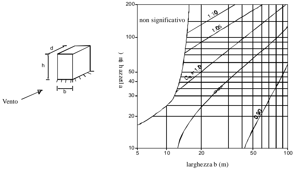
Fig. C.7.10 (b) - Edifici a struttura in acciaio
