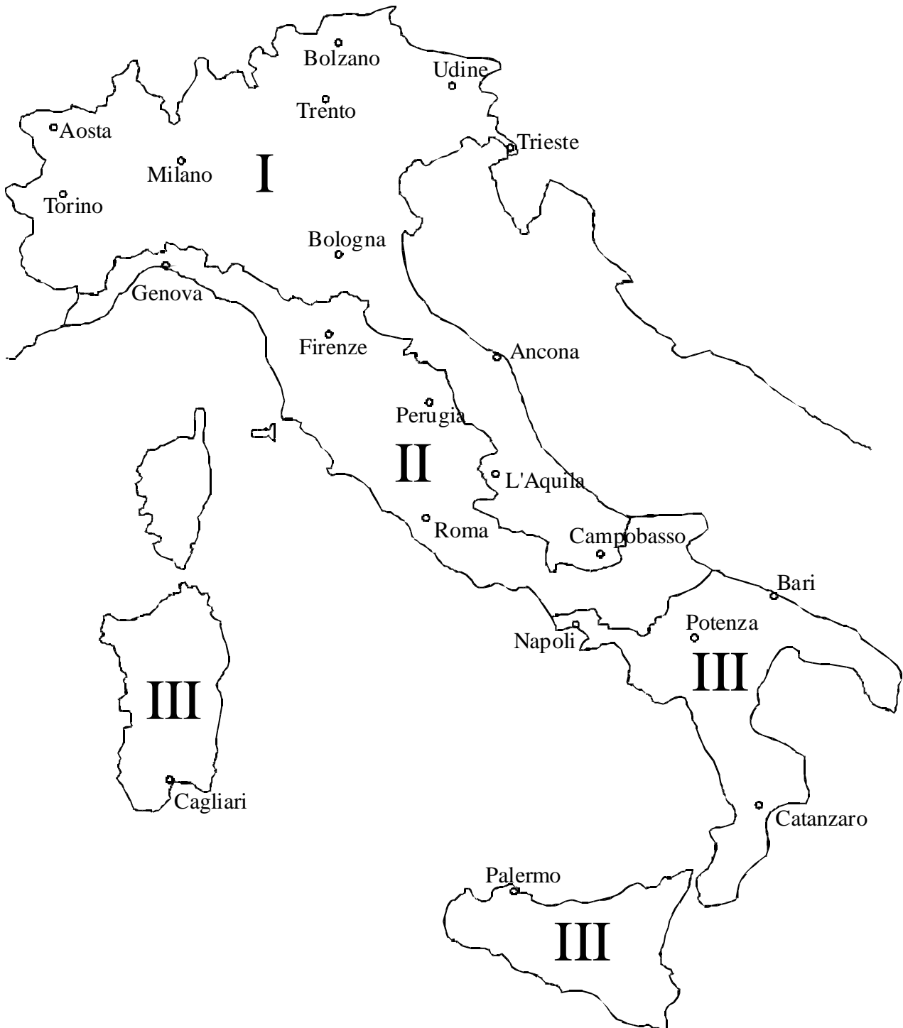
Fig. 6.1 - Mappa per carico neve al suolo
