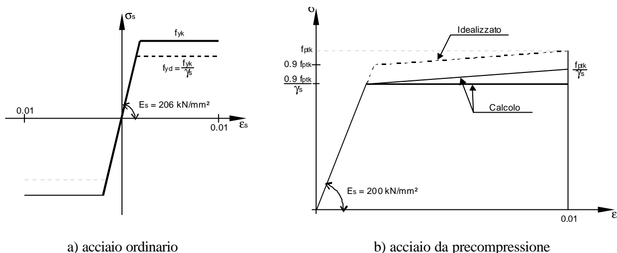
Fig. 3 - Diagramma di calcolo \sigma - \epsilon
