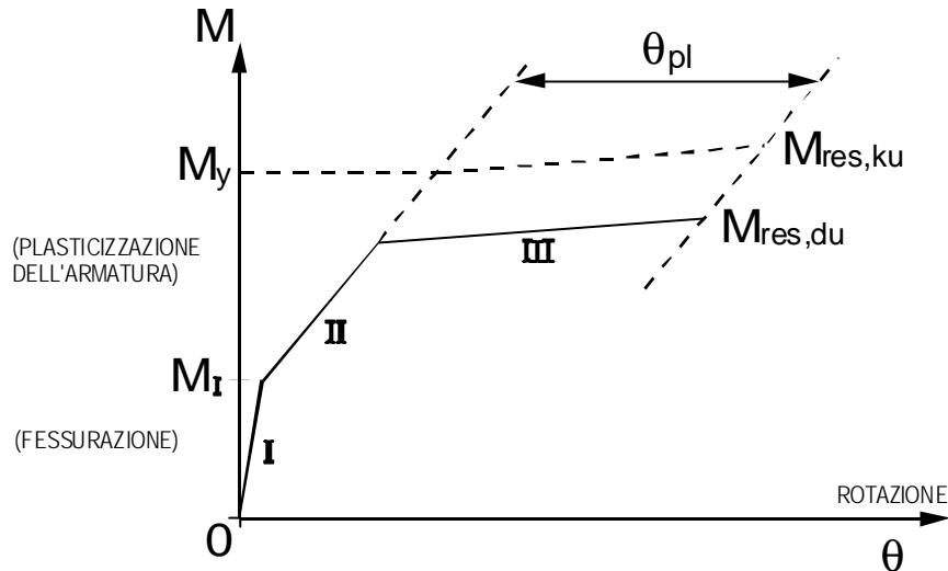
Fig. 1 - Diagramma momento-rotazione: idealizzazione tri-lineare
