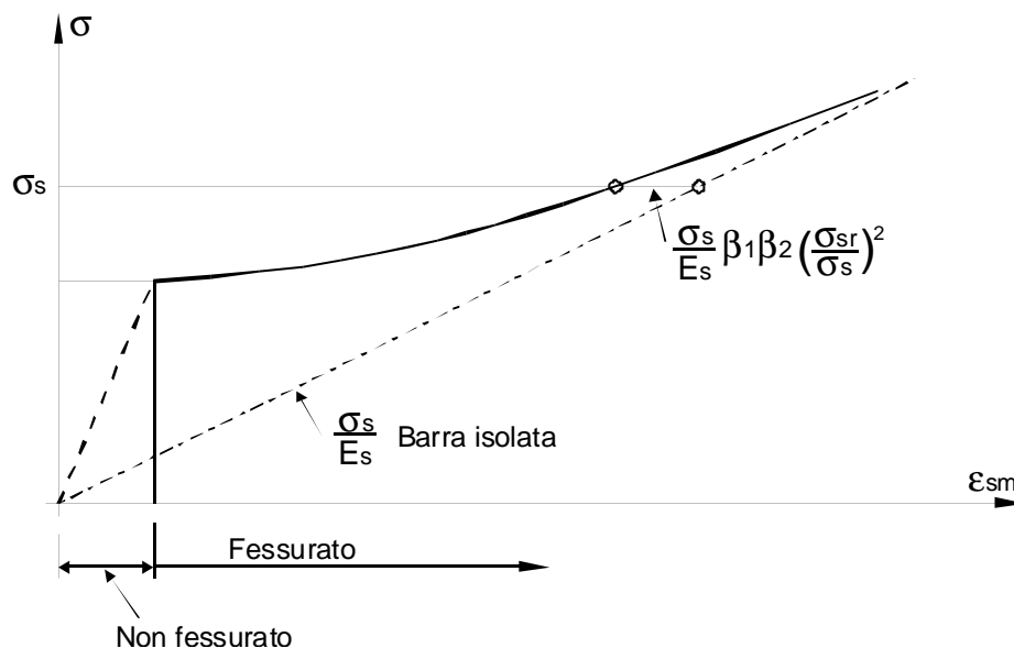
Fig. 5 - Diagramma \epsilon_{sm} - \sigma_s
