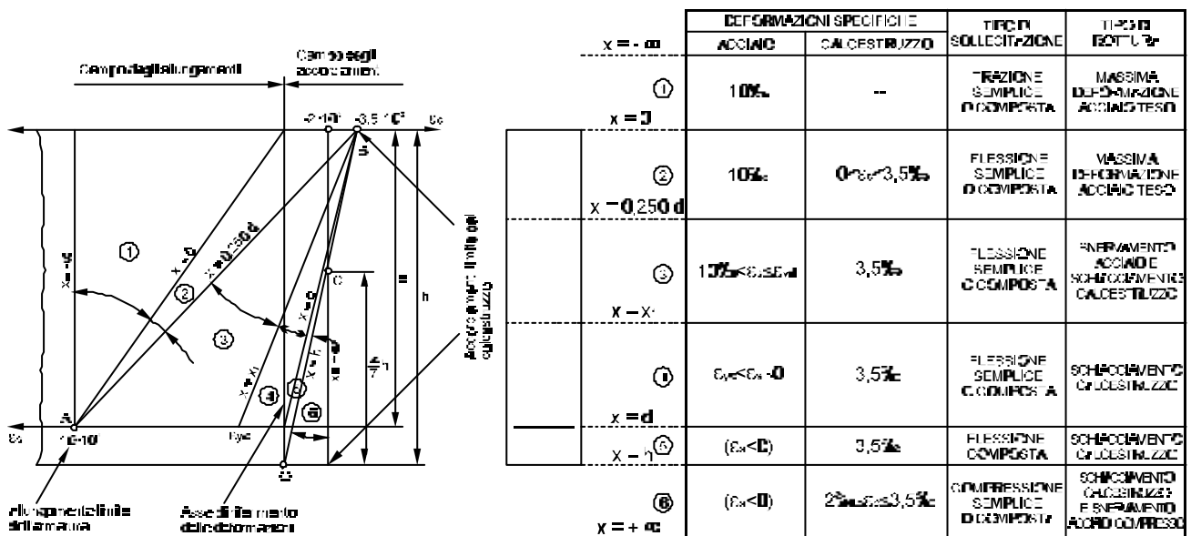
Fig. 2 - Diagramma di deformazione allo stato limite ultimo
