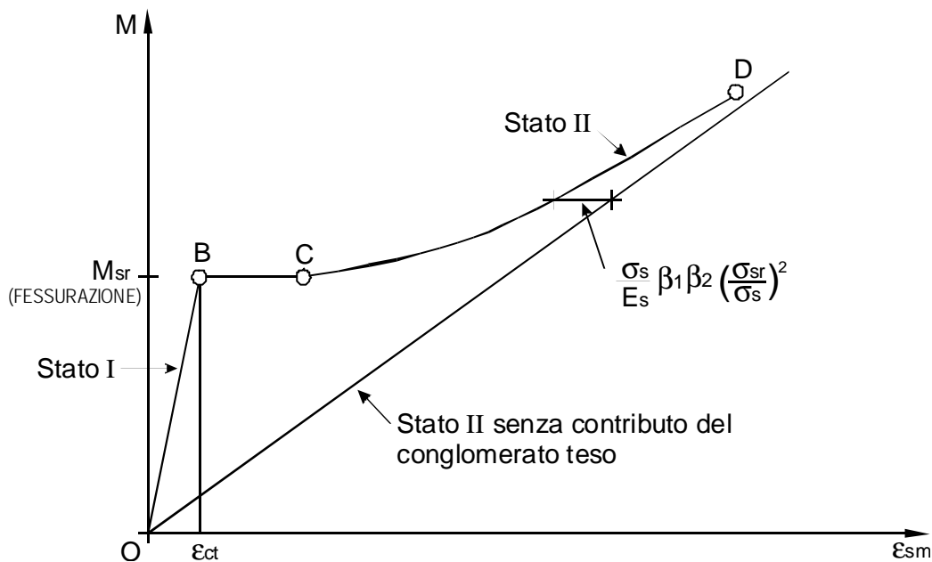
Fig. 6 - Diagramma M - \epsilon_{sm}
